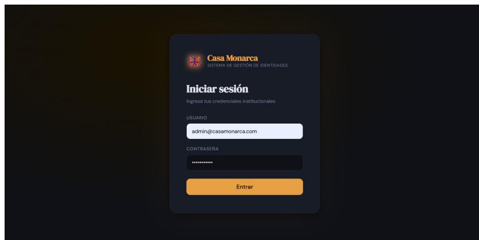
Figura 1: login - paso 1
